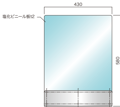
正面図
